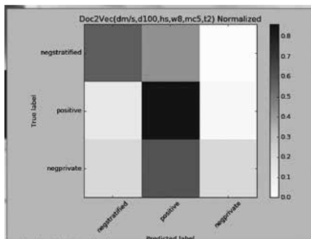
Рис. 5. Матрица неточностей для визуализации работы классификатора
